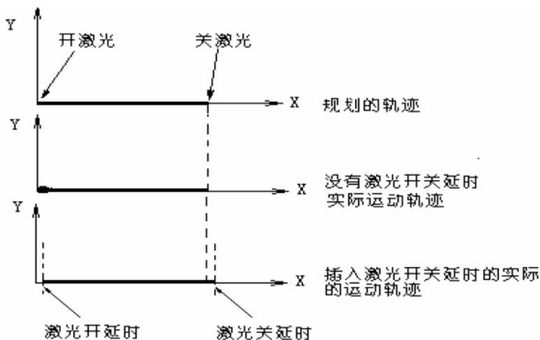
图 12-2-1 激光开关延时对轨迹的影响
